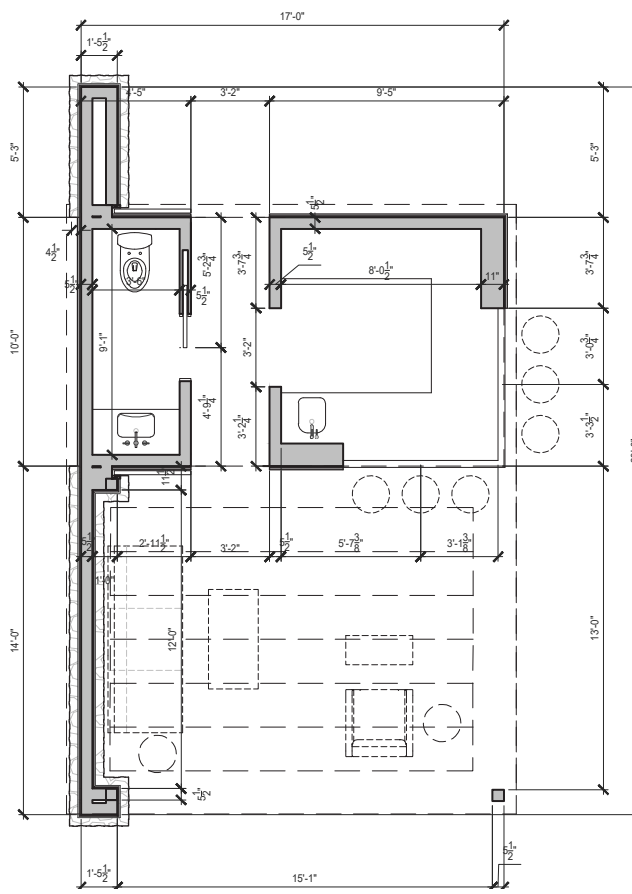
5 CABANA FLOOR PLAN SCALE: 1/8" = 1'
