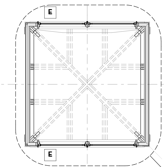
3 CUPOLA PLAN SCALE: 1/4" = 1'-0"
